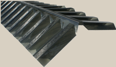
gop SUNTUF taknock. För anslutning av sadeltak. Längd: 1270 mm. Färg: klar och rök.
